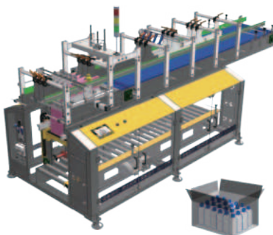
Машина для упаковки в картонные коробки
