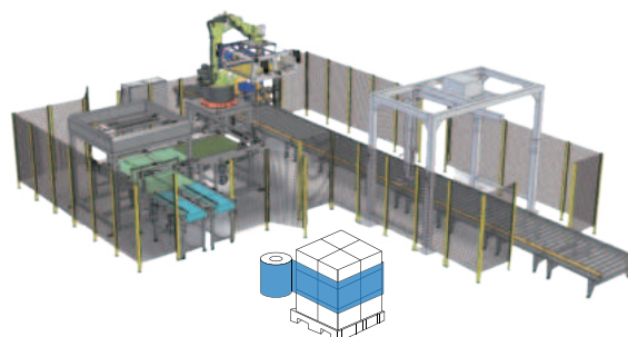
Паллетизатор + Палетообмотчик (стретч-плёнка)
