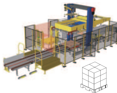
Депаллетизатор
